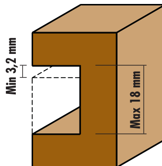
E182.476.R
