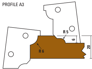
PROFILE A3
