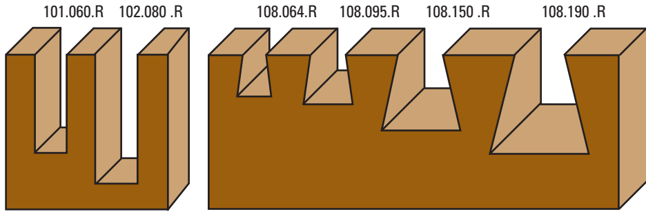
Scale 1:1
